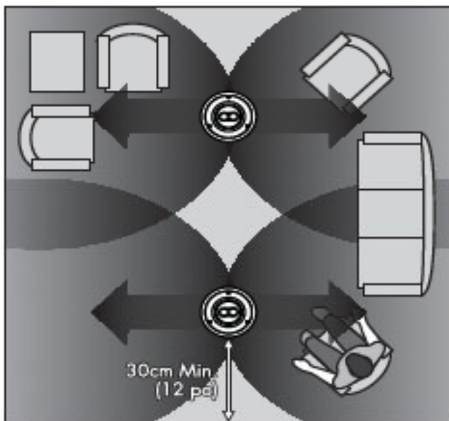
Figure 12. Helos 22: mode stéréo utilisé pour l'audio distribué.
