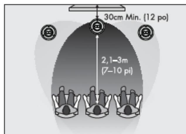
Figure 5. Helos 12: Ajouter un canal central.
