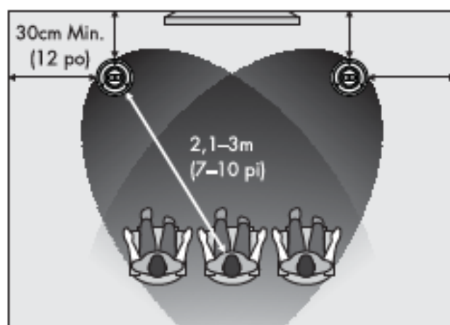
Figure 4. Helos 12: Installation à 2 canaux.
