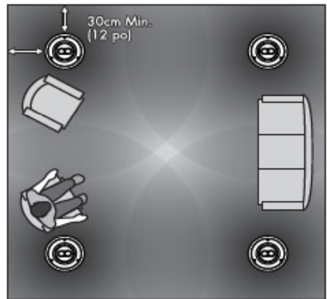
Figure 13. Helos 22: dispersion large. Mode mono utilisé pour l'audio distribué.
