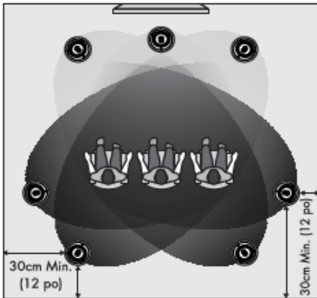
Figure 6. Helos 12: Ajouter des canaux ambiophoniques pour créer une installation à 5 ou 7 canaux.
